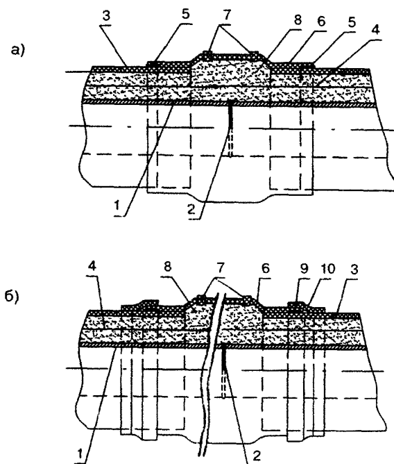
а - "сварка-заливка", б - "герметизация-заливка"
